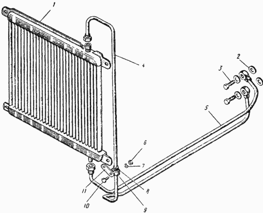
Рис. 29. Масляный радиатор
